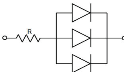
电路模式/ Circuit model B
